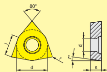
WCMT / WCMX
